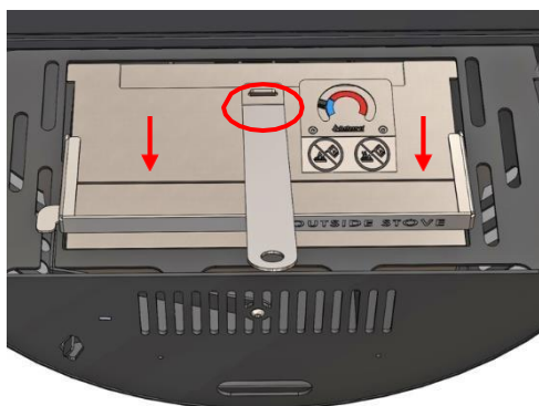
Obrázek 5 - Otevření hořáku pomocí rukojeti Aduro
