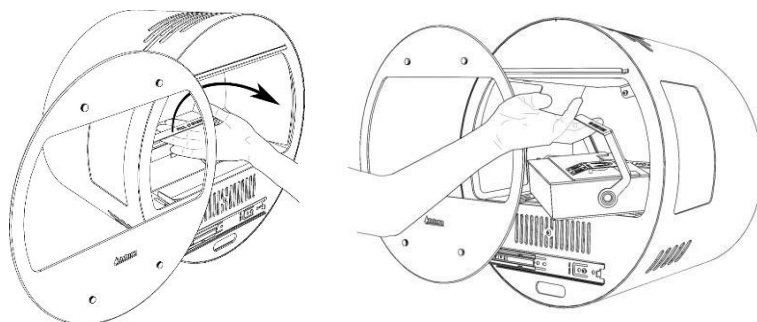
Obrázek 3 - Zvedněte rukojeť a vyjměte hořák
