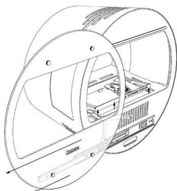
Obrázek 2 - Posuňte přední sklo na stranu
