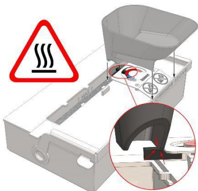
Obrázek 1 - Umístění nálevky Aduro
